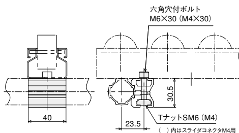
スライダコネクタ
