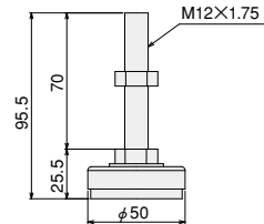
アジャスタA M12
