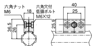
コネクタピース
