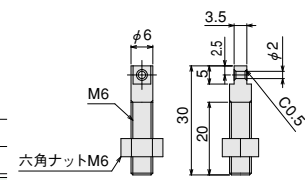
引張りバネポスト
