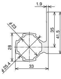
グリーンフレームF35
