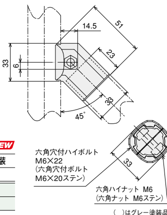
45°コネクタアウター型
