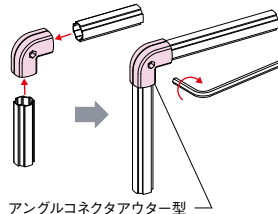
アングルコネクタアウター型
