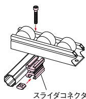
スライダコネクタ
