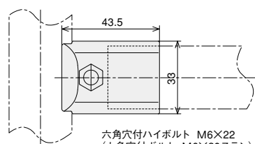
六角穴付ハイボルト M6×22 (六角穴付ボルト M6×20ステン)
