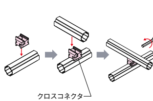
クロスコネクタ
