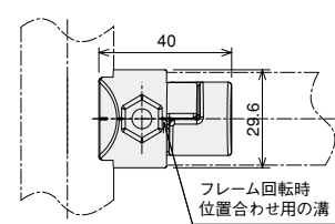
M6×18ボルト (六角穴付ボルト M6×18ステン)
