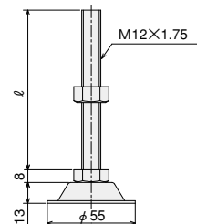
アジャスタB M12
