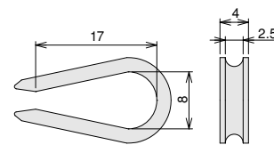
\phi 2 ワイヤーシンブル
