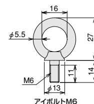
アイボルトM6
