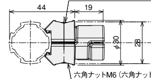
六角ナットM6 (六角ナット M6ステン) ( )はグレー塗装品
