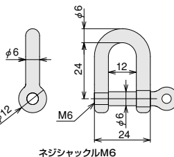
ネジシャックルM6
