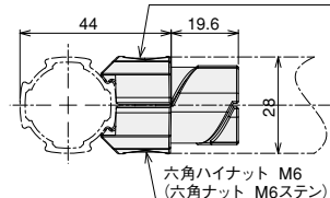
六角穴付ハイボルト M6×18 (六角穴付ボルト M6×18ステン)
