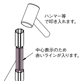
ストレートジョイント
