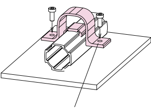
ダブルサドル
