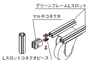
Lスロットコネクタピース
