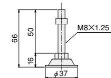
アジャスタB M8
