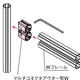
マルチコネクタアウター型W
