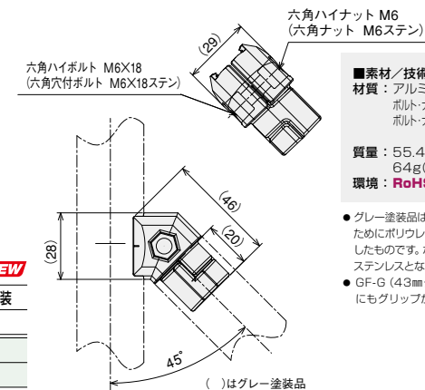
45°コネクタインナー型
