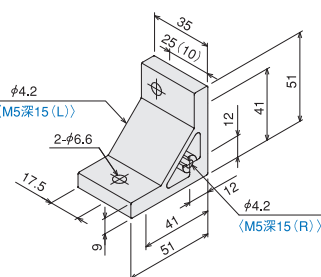
ハードブラケットL45-S・L(R)
