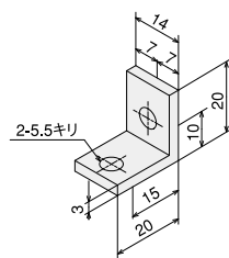
アングルブラケットSS
