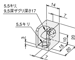
アングルブラケットハードSS
