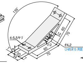
ハードブラケットSS2040・DE135
