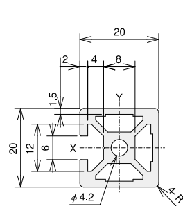
SF-20・20・3F
