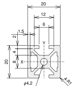
SF-20・20・2H
