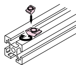
SフリーナットSS/アクセサリナットSS
