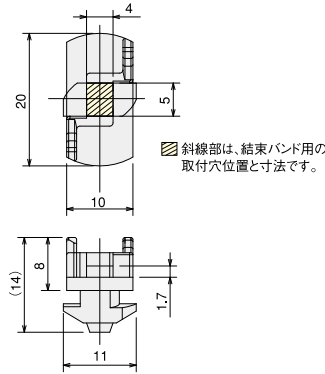
ケーブルクランプSS
