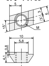
SフリーナットSS
