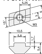
アクセサリナットSS(M3)
